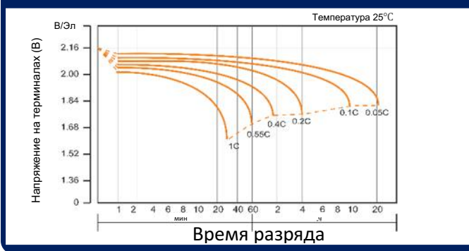
Кривые разряда
